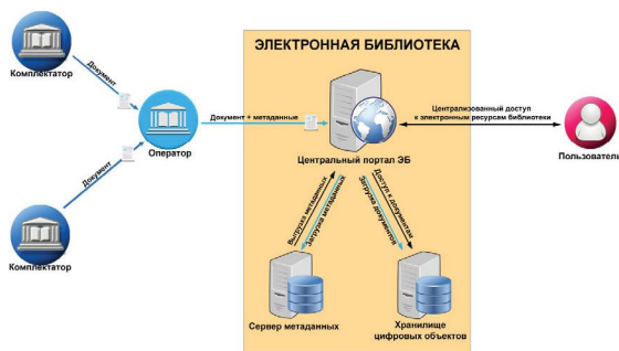
Рис. 2. Структура электронной библиотеки Fig. 2. The structure of the electronic library
